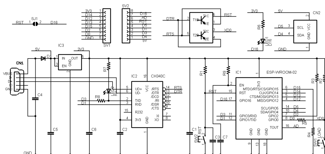
図 5.1 ESP8266-SLIM-R1 の回路図
