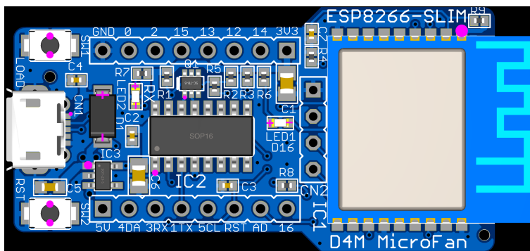
図 5.2 ESP8266-SLIM-R1 の部品配置
