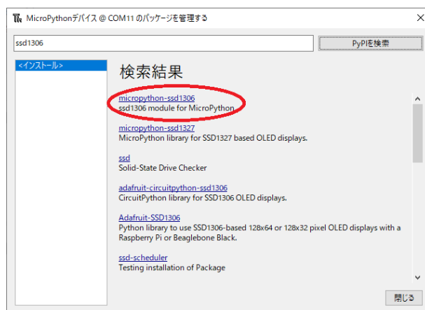
図 5.37 ssd1306 の検索
