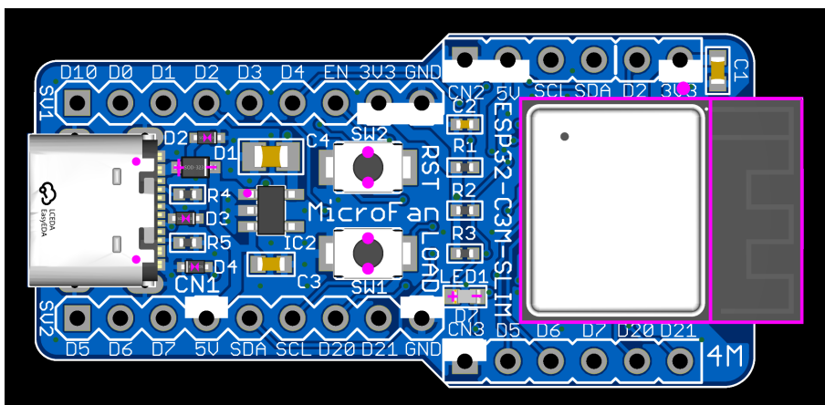
図 6.2 ESP32-C3M-SLIM-R1 の部品配置
