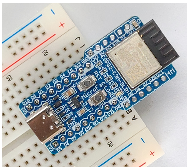
図 2.1 ブレッドボードに乗せた ESP32-C3M-SLIM-R1
