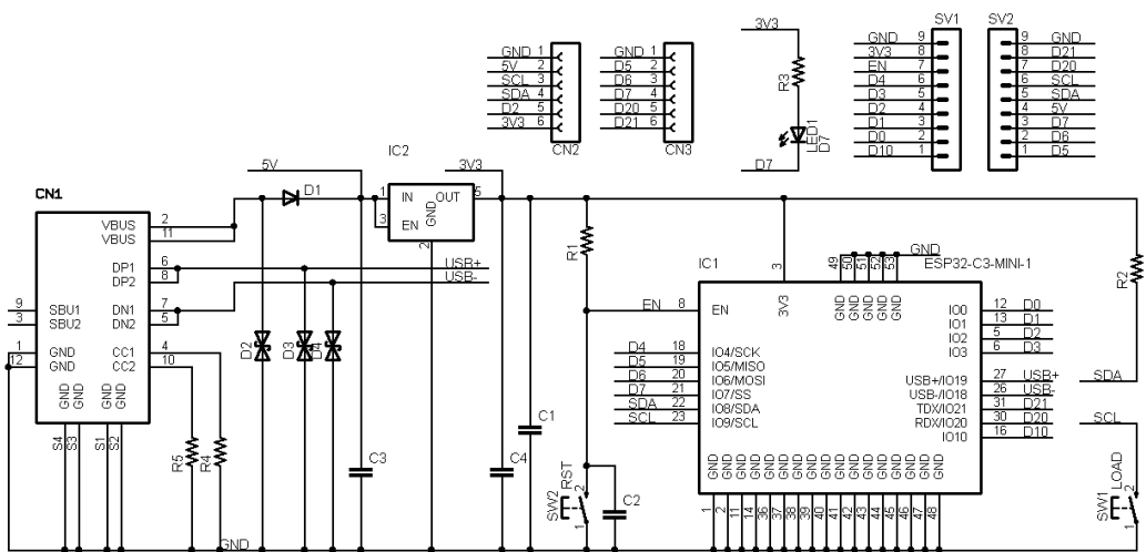
図 6.1 ESP32-C3M-SLIM-R1 の回路図
