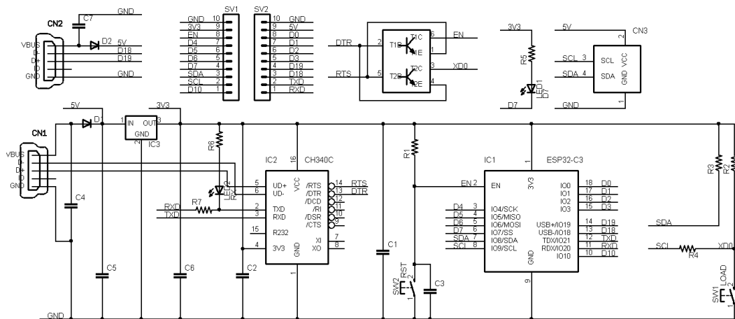
図 6.1 ESP32-C3-KEY-R1 の回路図
