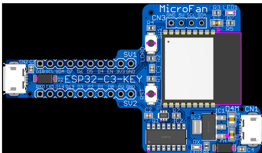
図 6.2 ESP32-C3-KEY-R1 の部品配置
