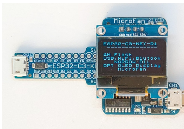
図 2.2 OLED ディスプレイを搭載した ESP32-C3-KEY-R1
