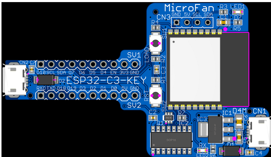
図 5.2 ESP32-C3-KEY-R1 の部品配置
