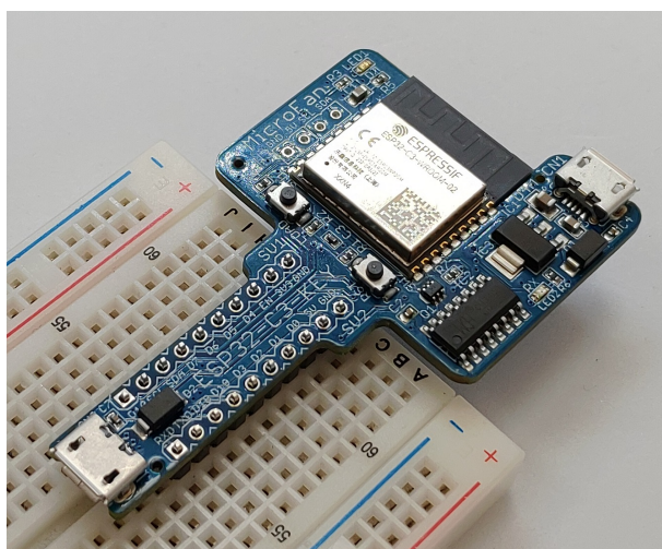
図 2.1 ブレッドボードに乗せた ESP32-C3-KEY-R1
