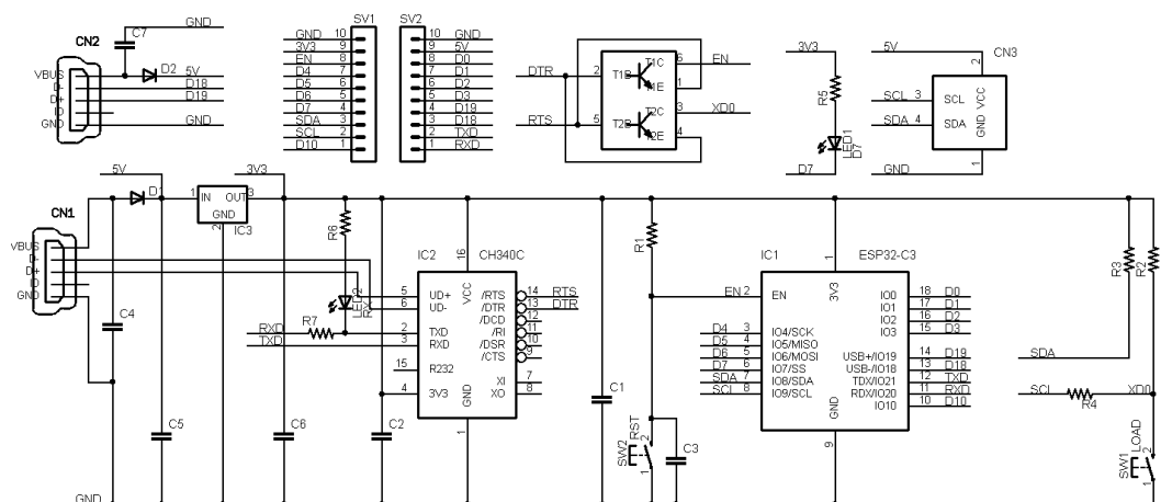
図 5.1 ESP32-C3-KEY-R1 の回路図
