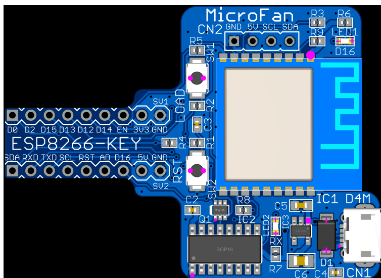
図 6.2 ESP8266-KEY-R2 の部品配置
