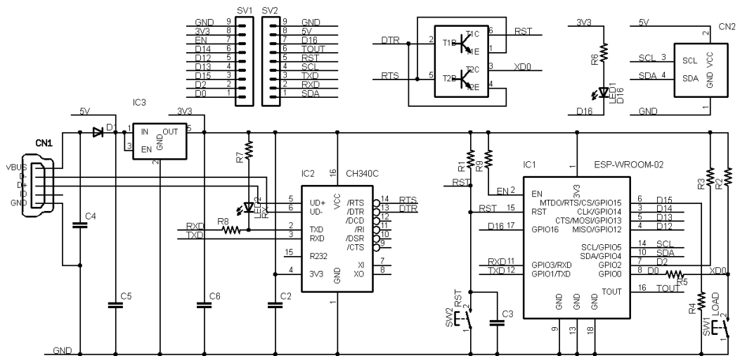
図 6.1 ESP8266-KEY-R2 の回路図
