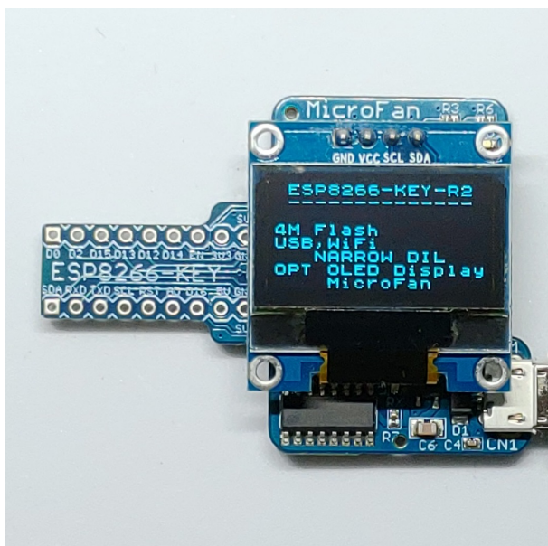
図 2.2 OLED ディスプレイを搭載した ESP8266-KEY-R2
