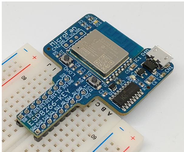
図 2.1 ブレッドボードに乗せた ESP8266-KEY-R2
