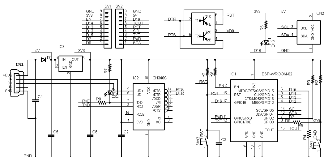
図 5.1 ESP8266-KEY-R2 の回路図
