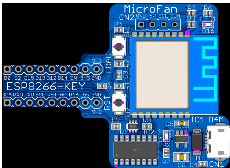
図 5.2 ESP8266-KEY-R2 の部品配置
