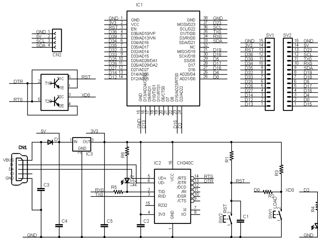
図 6.1 ESP32-KEY-R2 の回路図
