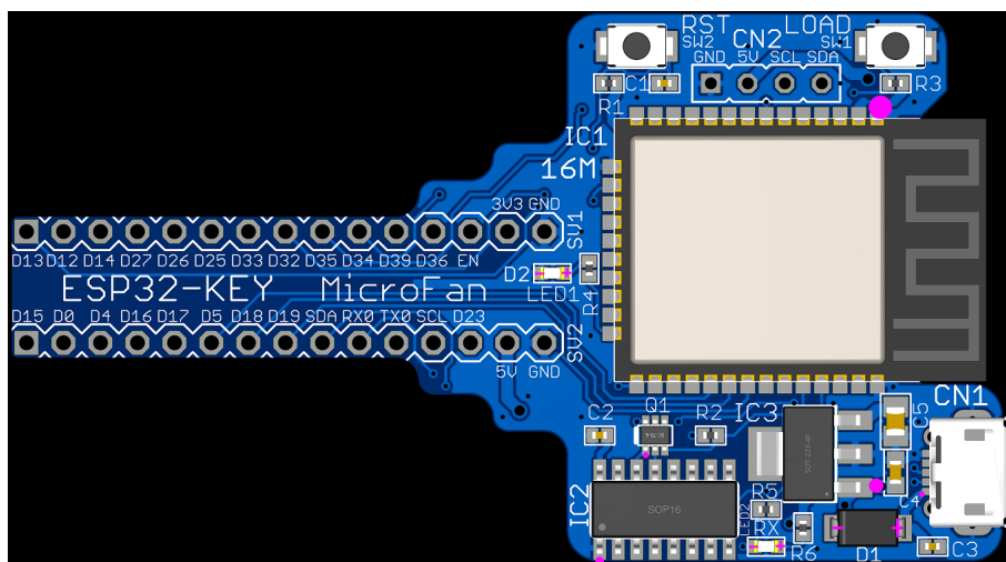
図 6.2 ESP32-KEY-R2 の部品配置
